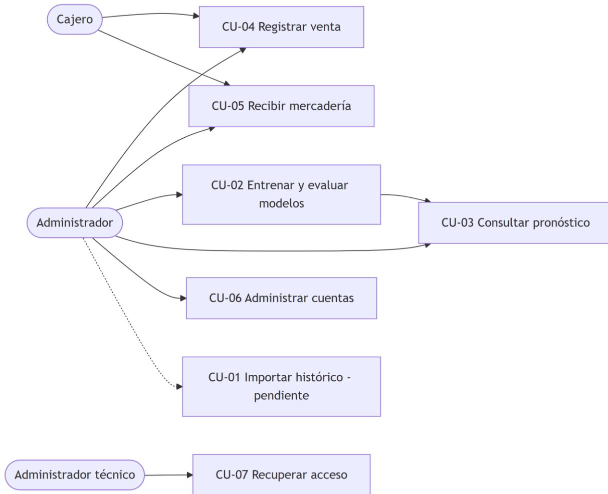
Figura 11. Diagrama de casos de uso del sistema. Fuente: Elaboración propia.
