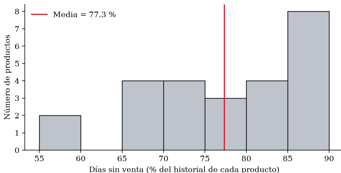
Figura 7. Distribución de la proporción de días sin venta por producto (n = 25). Fuente: Elaboración propia a partir de los registros del sistema (datos simulados).
