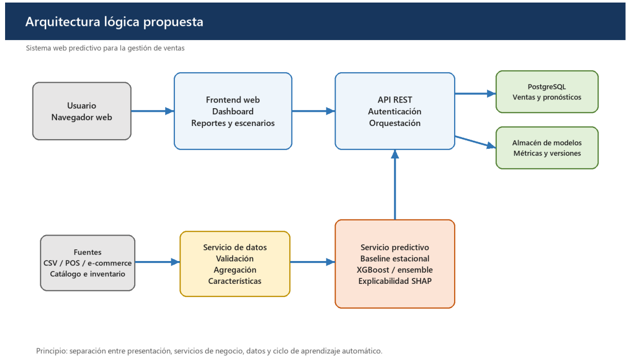
Figura 1. Arquitectura lógica propuesta para el sistema. Fuente: Elaboración propia.
