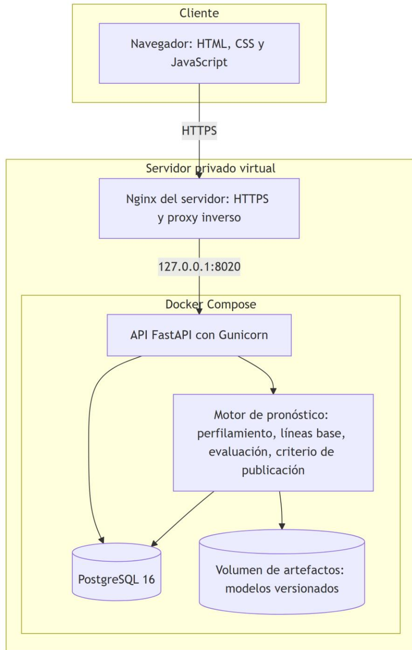
Figura 12. Arquitectura desplegada de la solución. Fuente: Elaboración propia.
