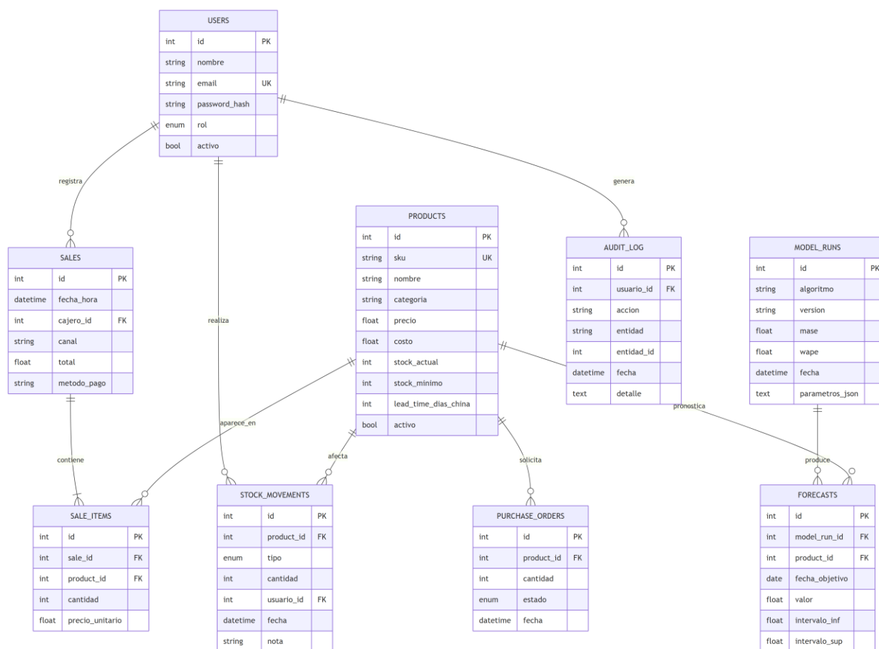
Figura 13. Modelo entidad-relación implementado. Fuente: Elaboración propia.
