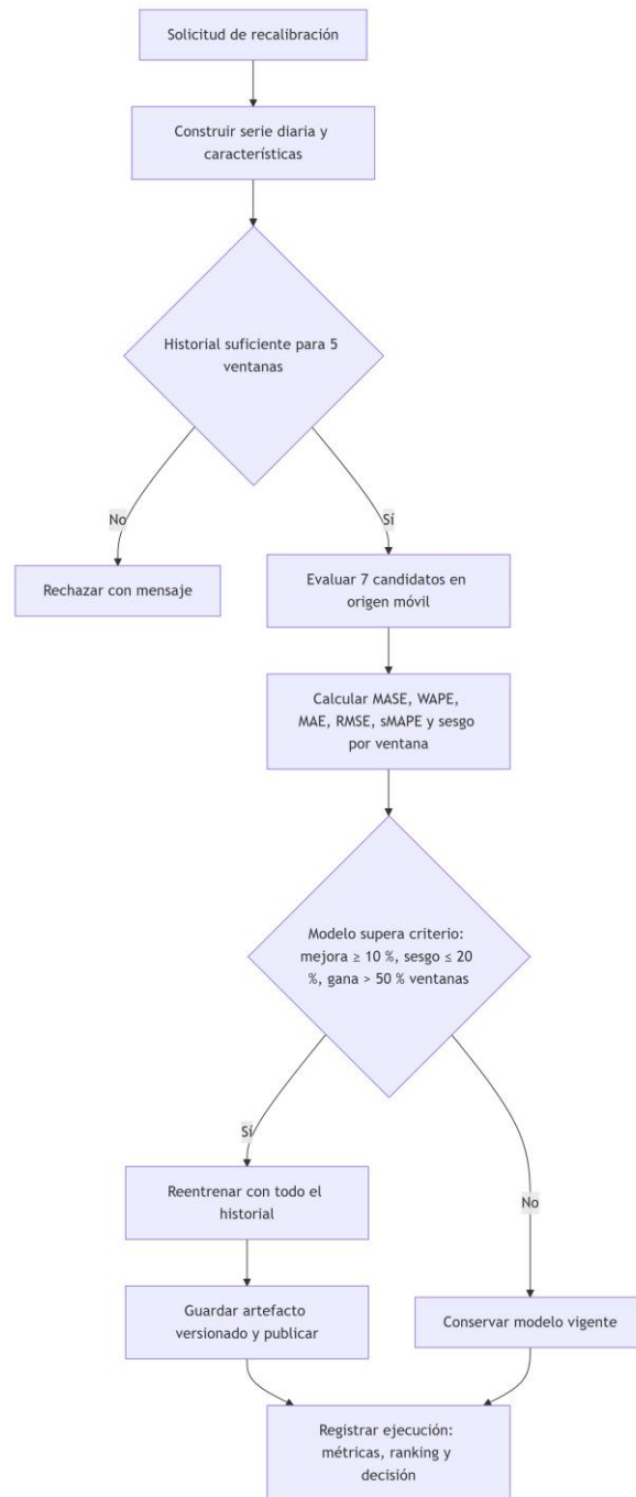
Figura 14. Flujo de una recalibración del modelo. Fuente: Elaboración propia.
