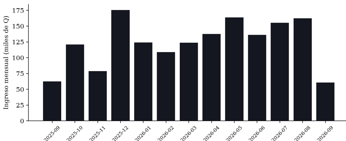
Figura 9. Ingreso mensual simulado. Fuente: Elaboración propia a partir de los registros del sistema (datos simulados).
