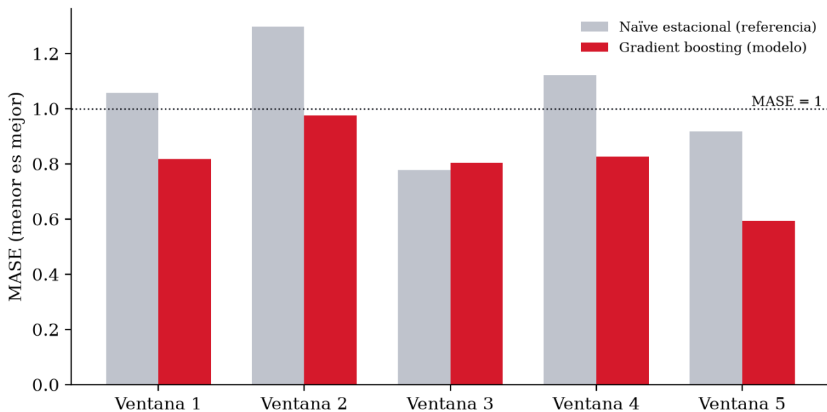
Figura 10. MASE por ventana de validación: modelo frente a la referencia naïve estacional. Fuente: Elaboración propia a partir de los registros del sistema (datos simulados).
