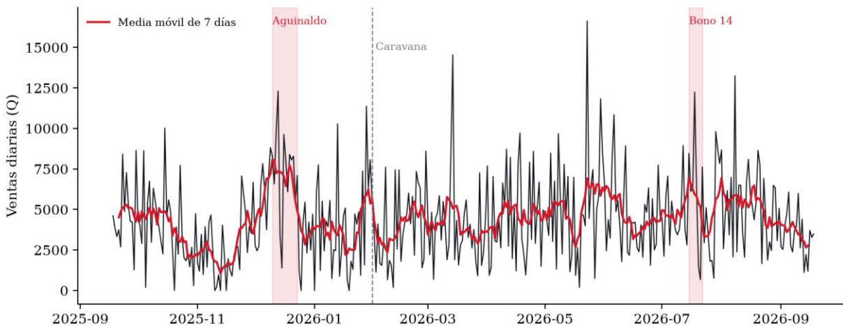
Figura 8. Serie diaria simulada de ventas con los periodos de temporada alta señalados.
